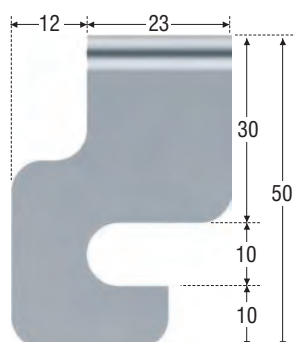
Вид сбоку
