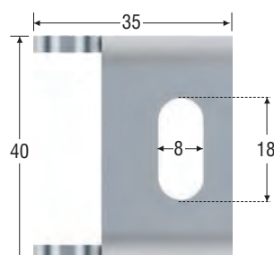
Вид сверху
